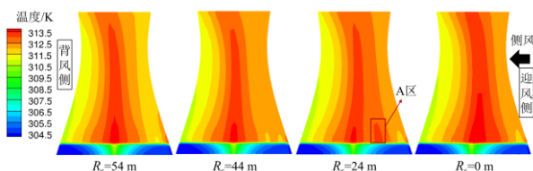
图 11 不同扇区内径下冷却塔内空气温度场云图 ( X=0 m)
