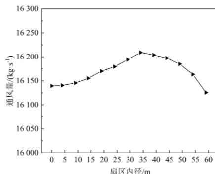
a) 通风量随扇区内径的变化曲线
